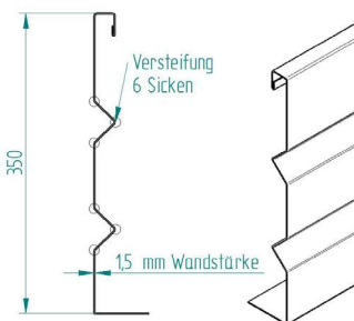
Wandprofil verstärkte Ausführung
