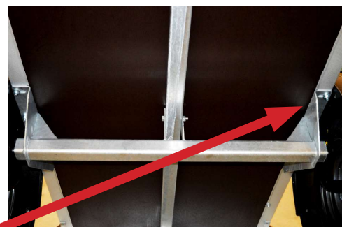
500mm Achsauflage und Knotenblechversteifung
